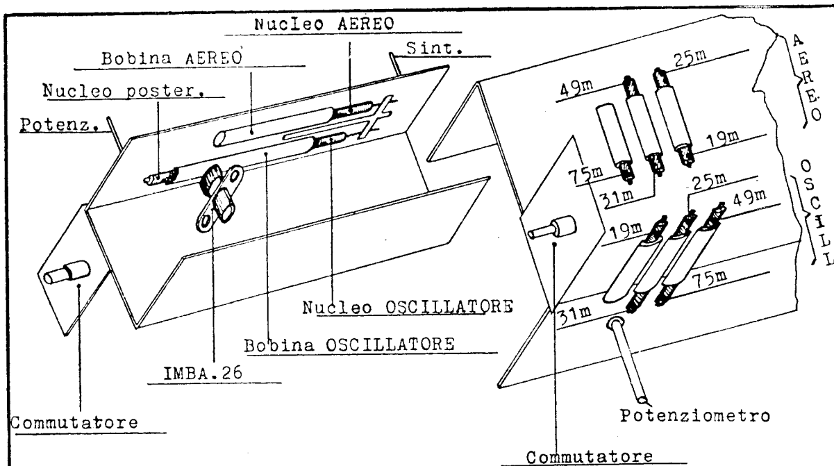
Apparecchio R. 56/2 con A.F. 62/3 PV
